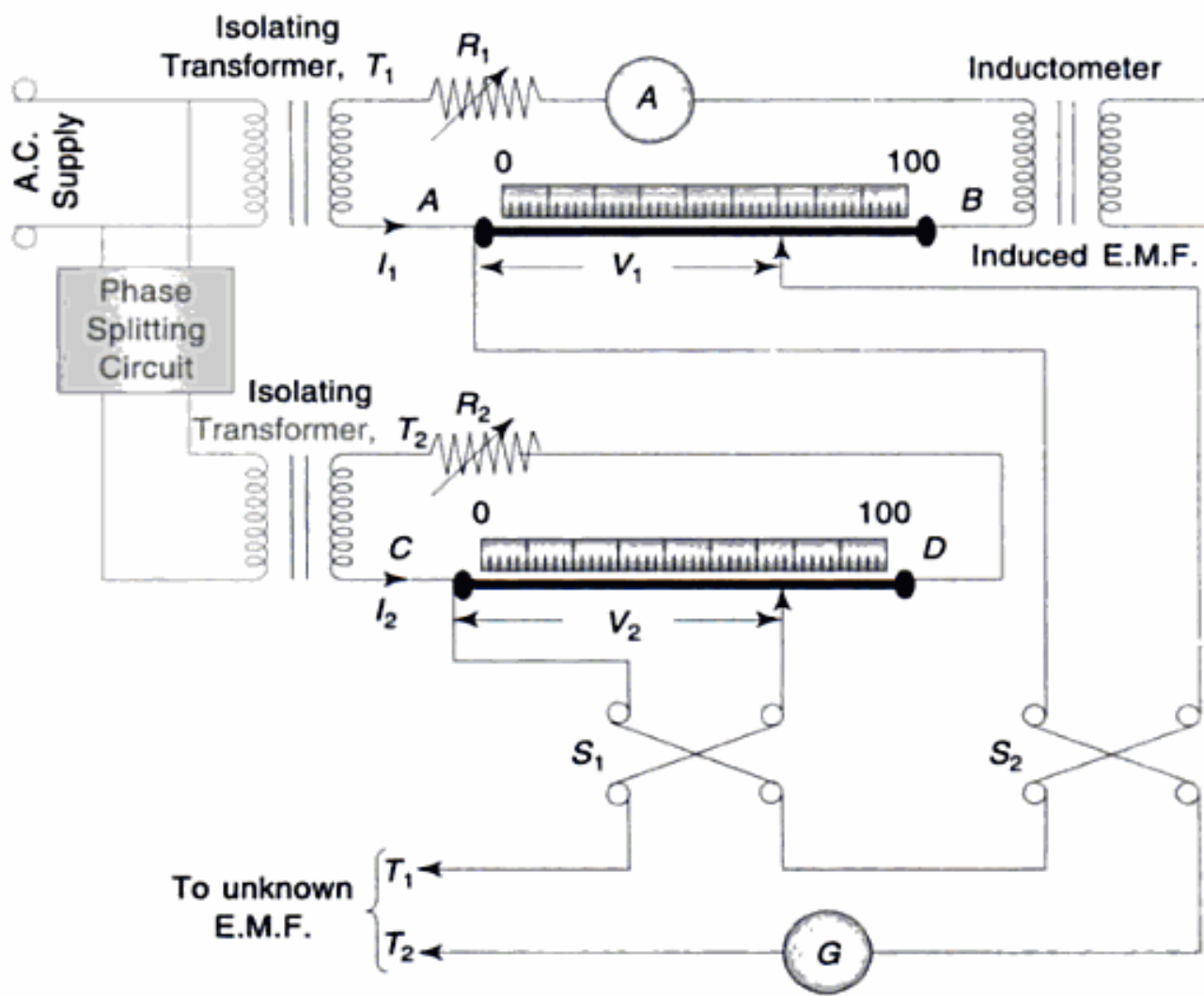
Fig. 2.38 Gall-Tinsley Potentiometer
