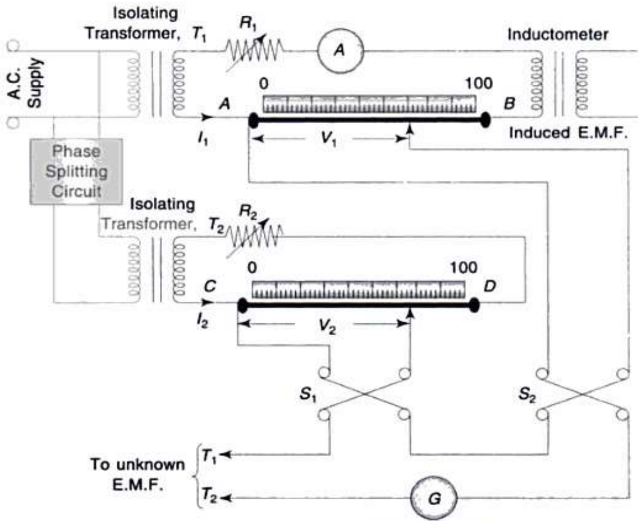
Fig. 2.38 Gall-Tinsley Potentiometer
