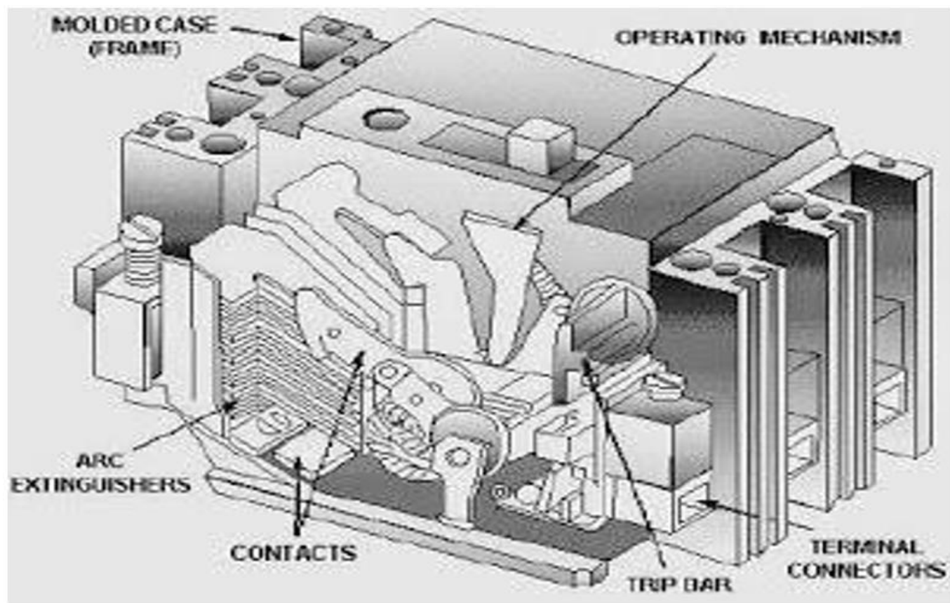
MCCB
